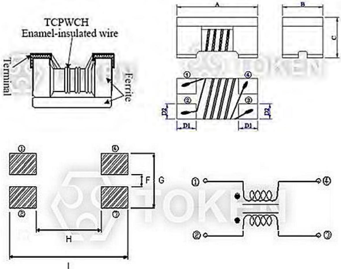
共模濾波器車規 (TCPWCH-4532AU) 結構圖 單位: mm (Inch)
