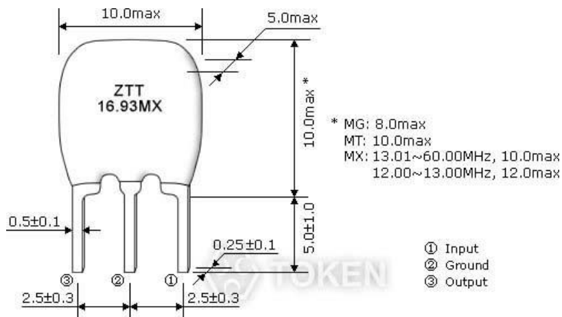
(ZTT16.93MX) Dimensions
