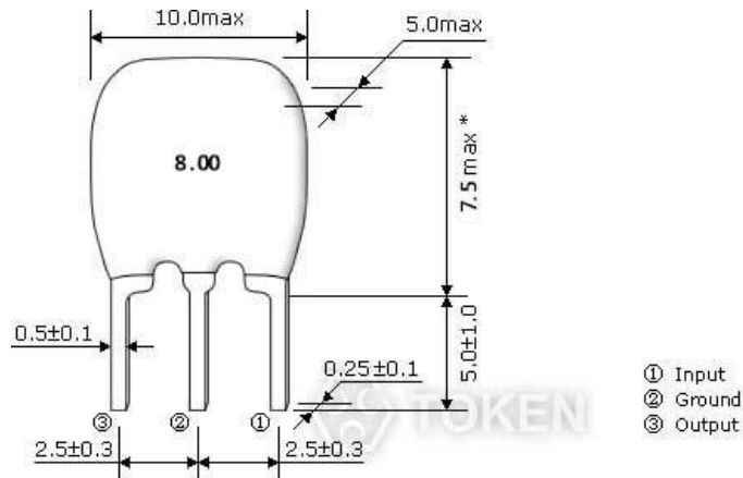
(ZTTLS8.00MG) Dimensions
