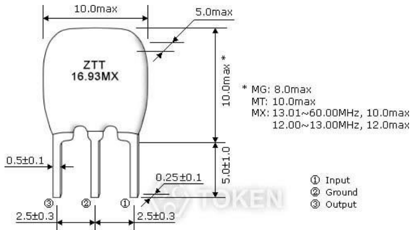
(ZTT16.93MX) Dimensions
