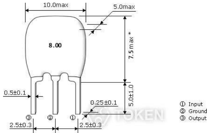
(ZTTLS8.00MG) Dimensions
