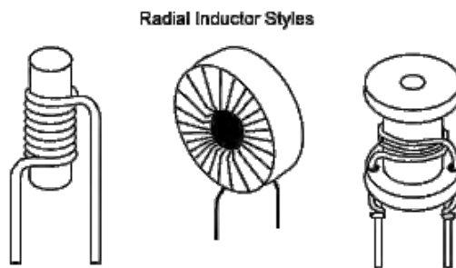
徑向電感的形式：棒形、環形、線軸形
