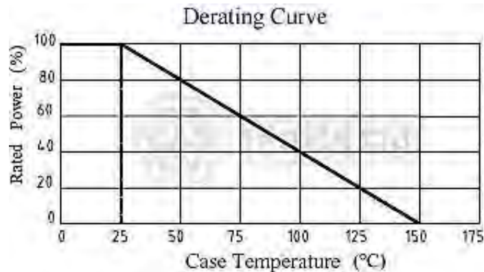
TO-220 功率電阻 (RMG50) 降額曲線
