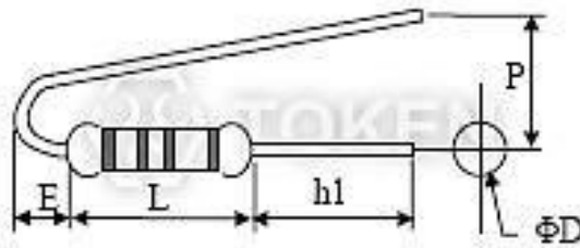
引腳加工成形 - F 型電阻尺寸
