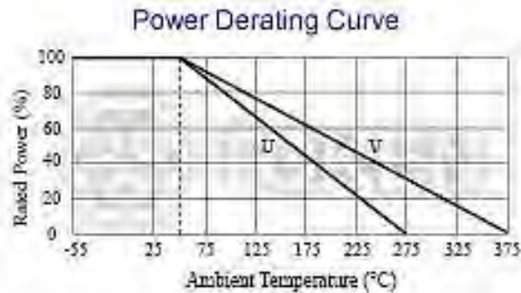
精密繞線電阻器 (KNP-R) 降額功率曲線圖
