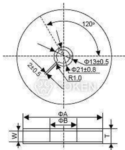
(TA7C/6C/5C/4C) Reel Dimensions
