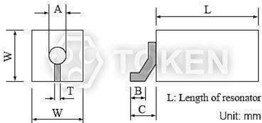
(DR) Dimensions
